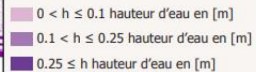
Carte de l'aléa de ruissellement (OFEV, 2018)
