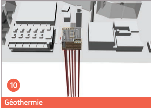
Géothermie Source d'énergie principale du réseau de chaleur à distance et anergie du quartier Bluefactory
