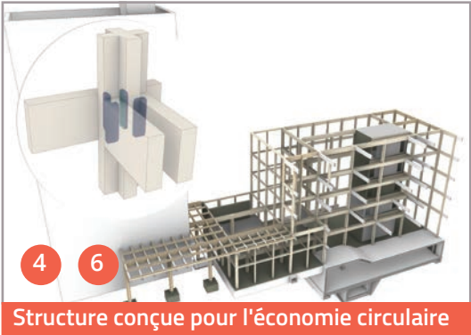
Structure conçue pour l'économie circulaire Système structurel composé d'éléments préfabriqués en bois local permettant une réutilisation en fin de vie du bâtiment
