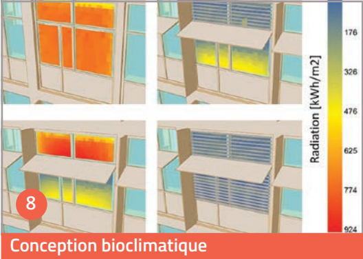
Conception bioclimatique Gestion du confort hygrothermique par des stratégies passives comme les protections solaires mobiles et la ventilation naturelle circulant entre les jardins d'hiver et l'atrium central
