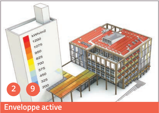
Enveloppe active Irradiation solaire annuelle cumulée sur les modules de l'installation photovoltaïque intégrée à l'enveloppe du bâtiment
